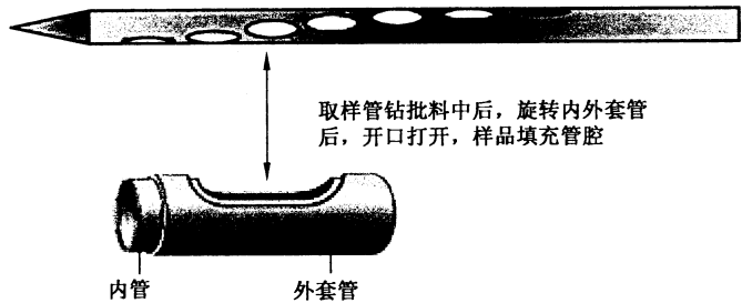
图 6 取样管示意图
