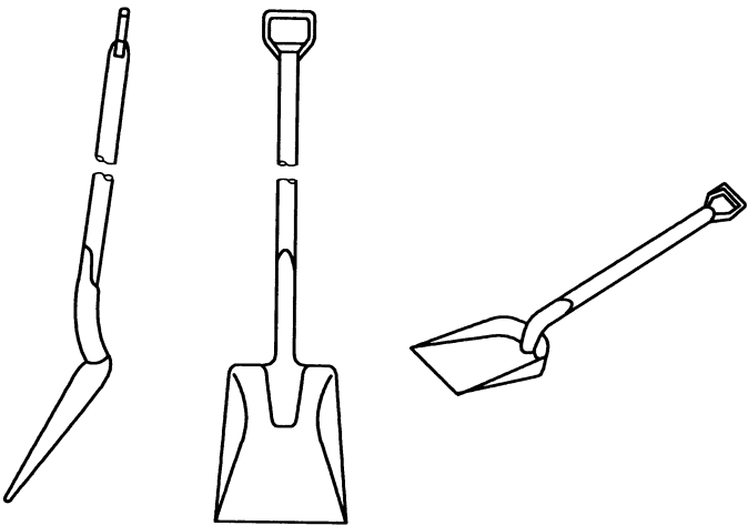
图 3 平底铲示意图
