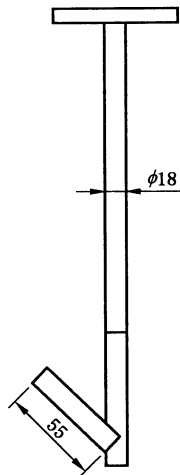
图 5 高长径比材料(秸秆)取样钩的示意图
