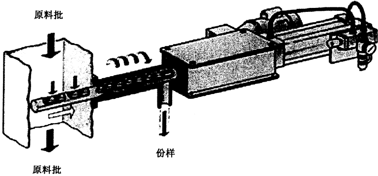
图 9 螺杆落流取样机
