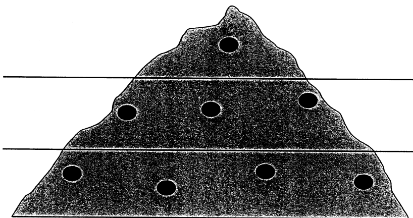
图 10 小料堆的采样点分布示意图
