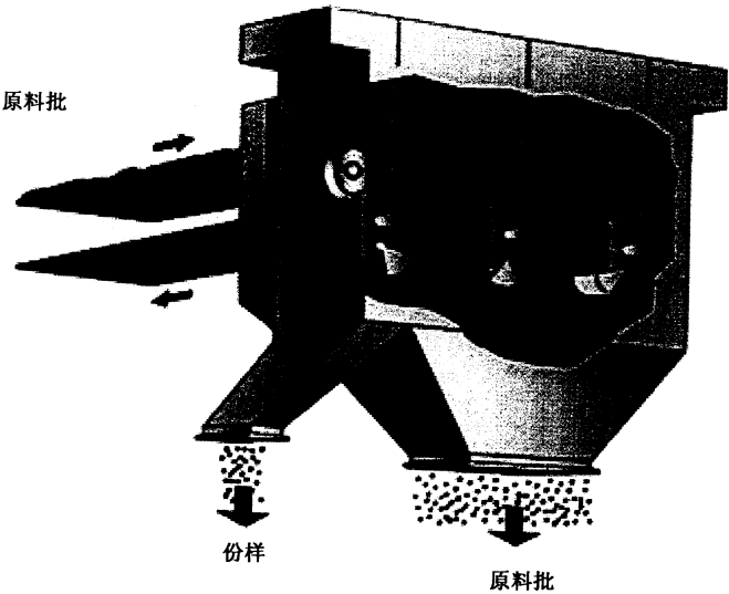
图 7 传输带截面取料机
