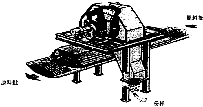
图 7 传输带截面取料机
